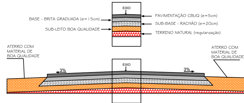
SEÇÃO TIPO PAVIMENTAÇÃO SEM ESCALA
