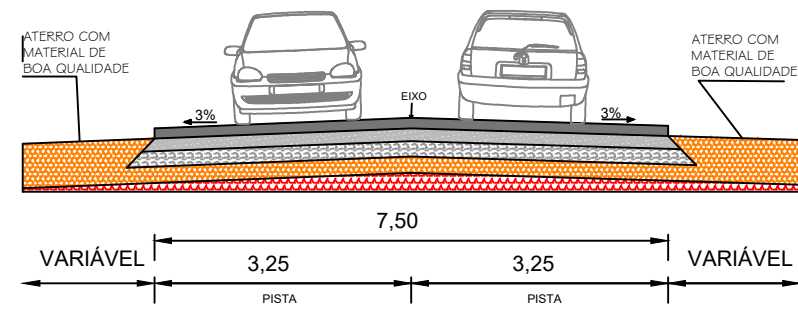
SEÇÃO TIPO PAVIMENTAÇÃO SEM ESCALA
