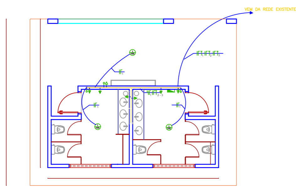
PLANTA BAIXA - ELÉTRICO ESCALA 1/75
