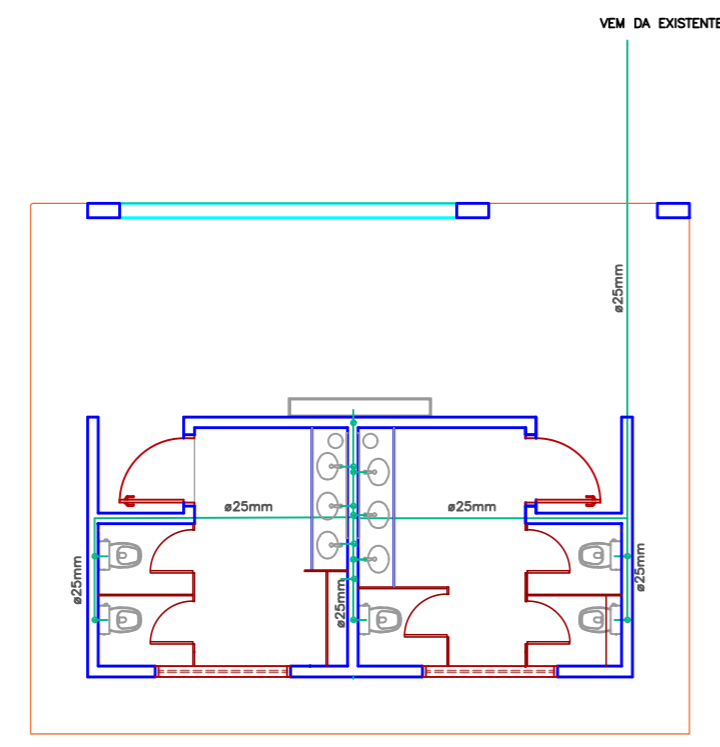
PLANTA BAIXA - HIDRÁULICO ESCALA 1/75
