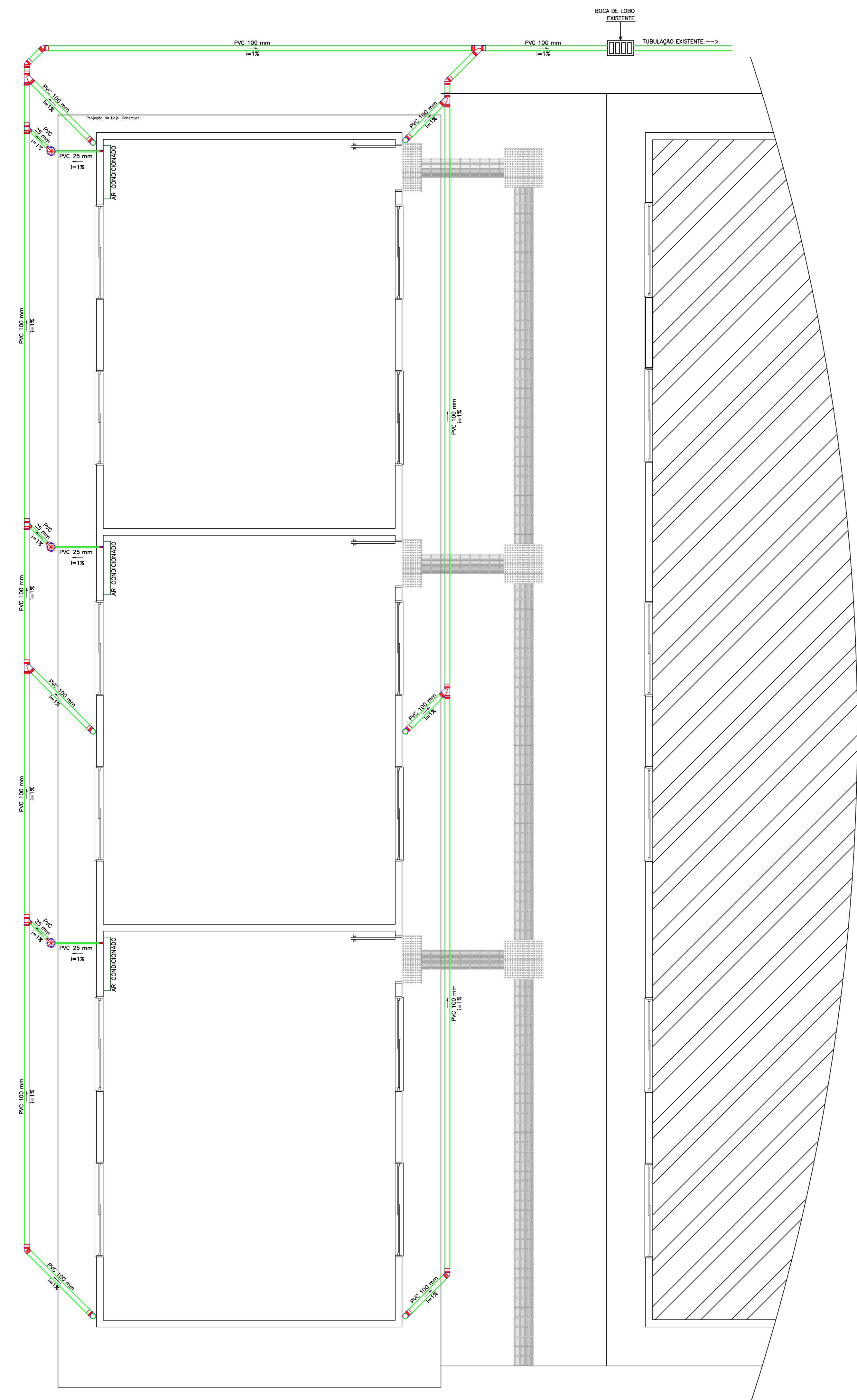
PLANTA DO SISTEMA DE DRENAGEM PLUVIAL ESC. 1/50
