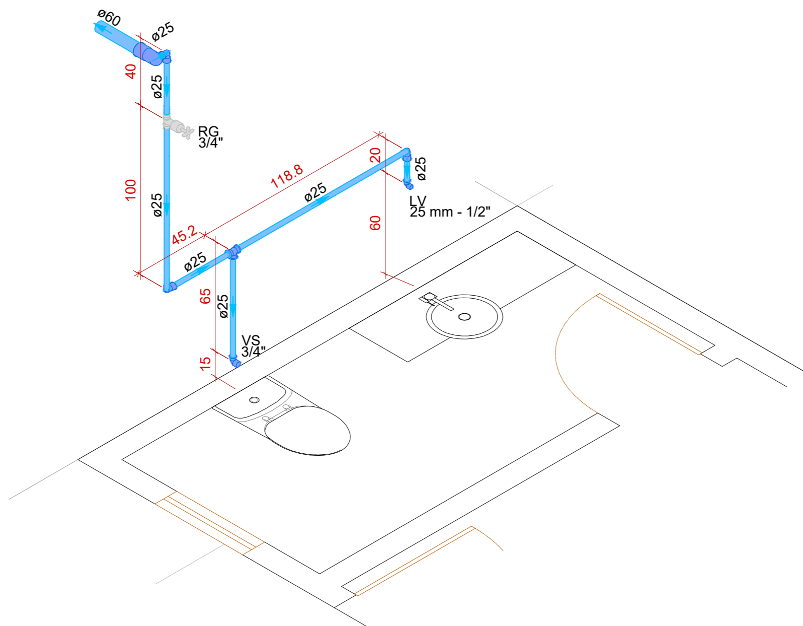
Detalhe Isométrico (HID-1) Lavabo Escala: 1:75
